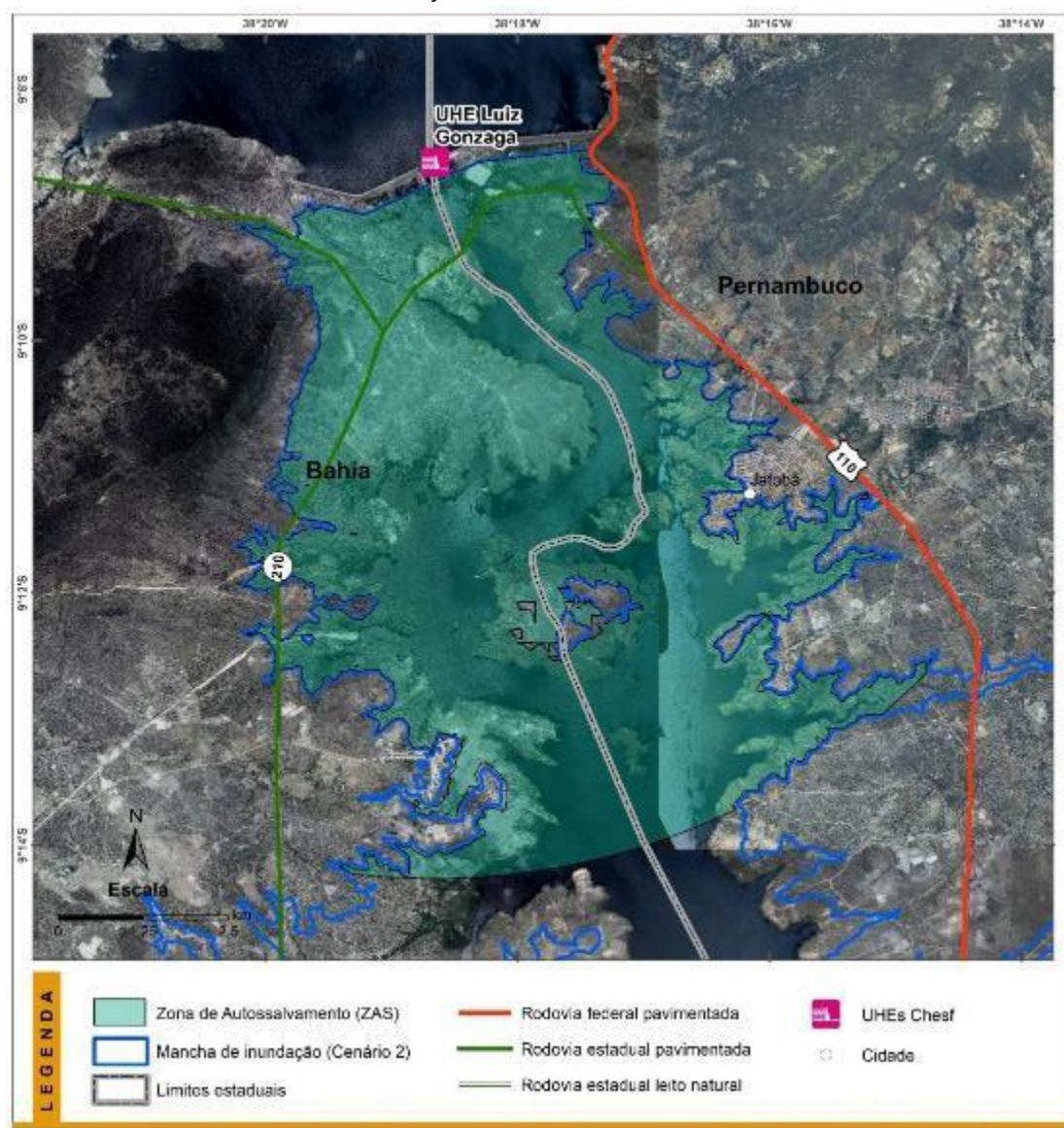
FIGURA 6.1 – IDENTIFICAÇÃO DA ZONA DE AUTOSSALVAMENTO – ZAS
