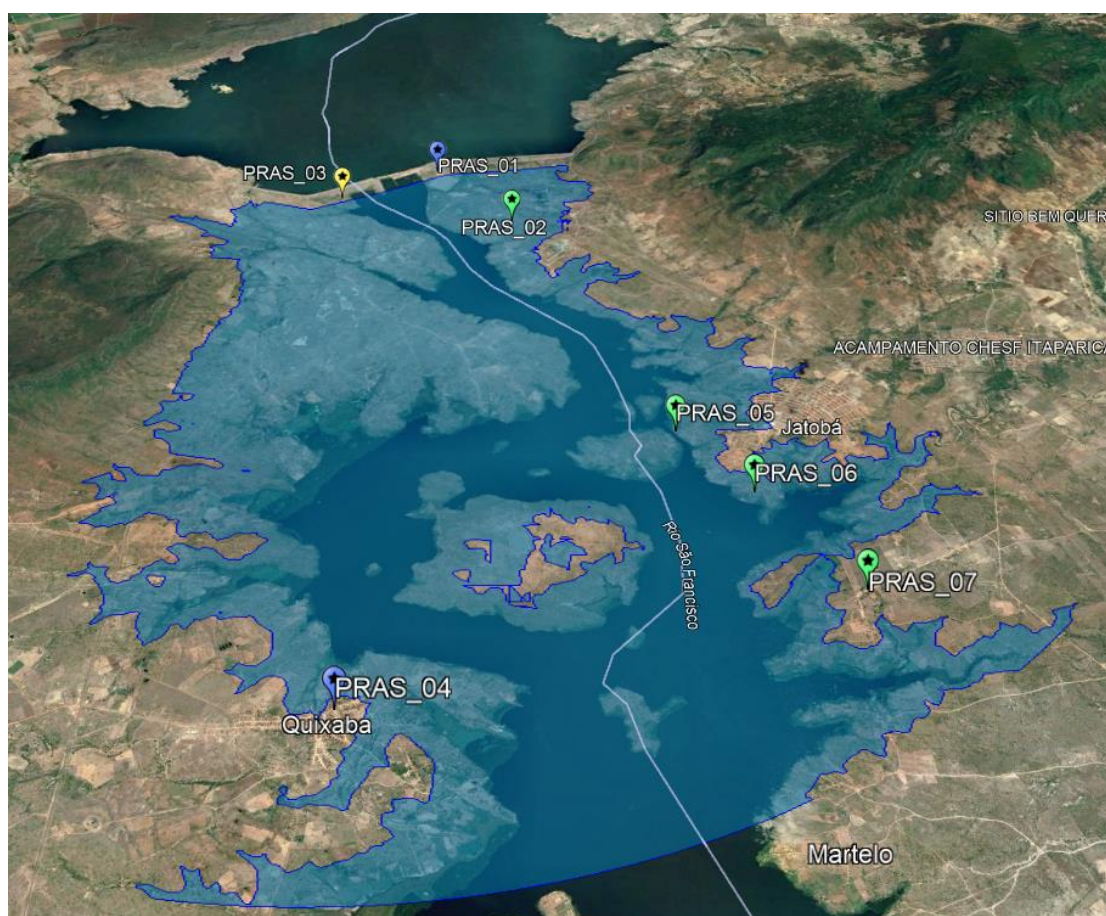
FIGURA 8.1 – LOCALIZAÇÃO DAS SIRENES
