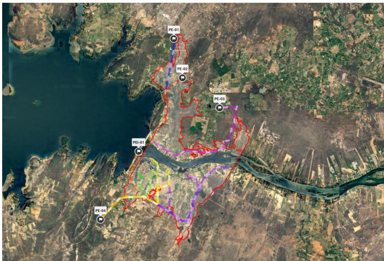
FIGURA 10.1 – ROTAS DE FUGA E PONTOS DE ENCONTRO NA ZAS DA UHE SOBRADINHO NOS MUNICÍPIOS DE PETROLINA E SOBRADINHO
