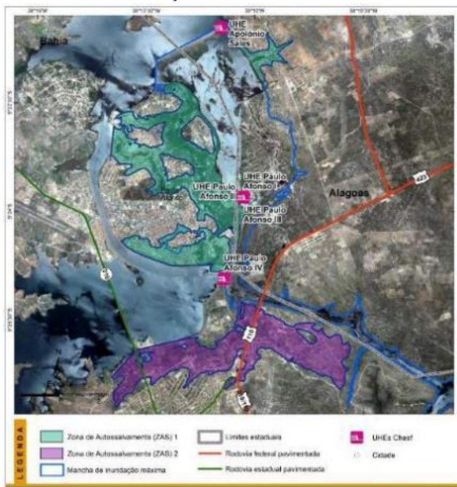
FIGURA 6.1 – IDENTIFICAÇÃO DA ZONA DE AUTOSSALVAMENTO – ZAS
